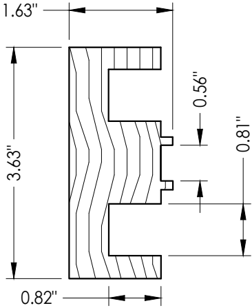
3 JAMB
